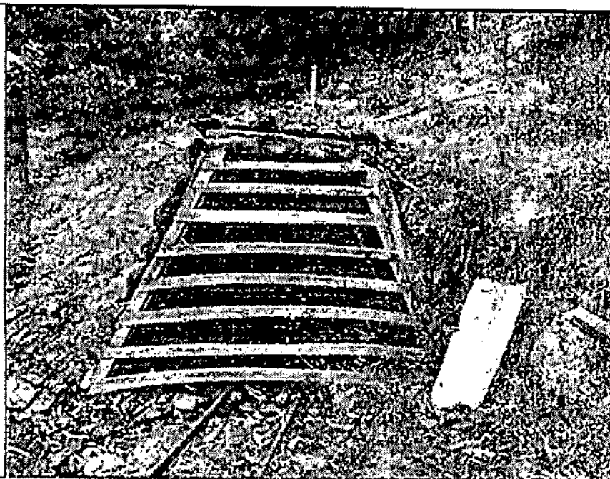
Fotografía No. 4. Bocamina inactiva denominada JACOBO, con las siguientes Coordenadas 1.025.201 Norte: 1.067.174 Altura: 2936 m.s.n.m.
