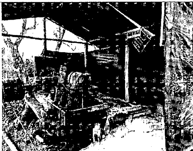
Fotografía No. 3. Instalaciones correspondientes a la Bocamina LA BACANA.
